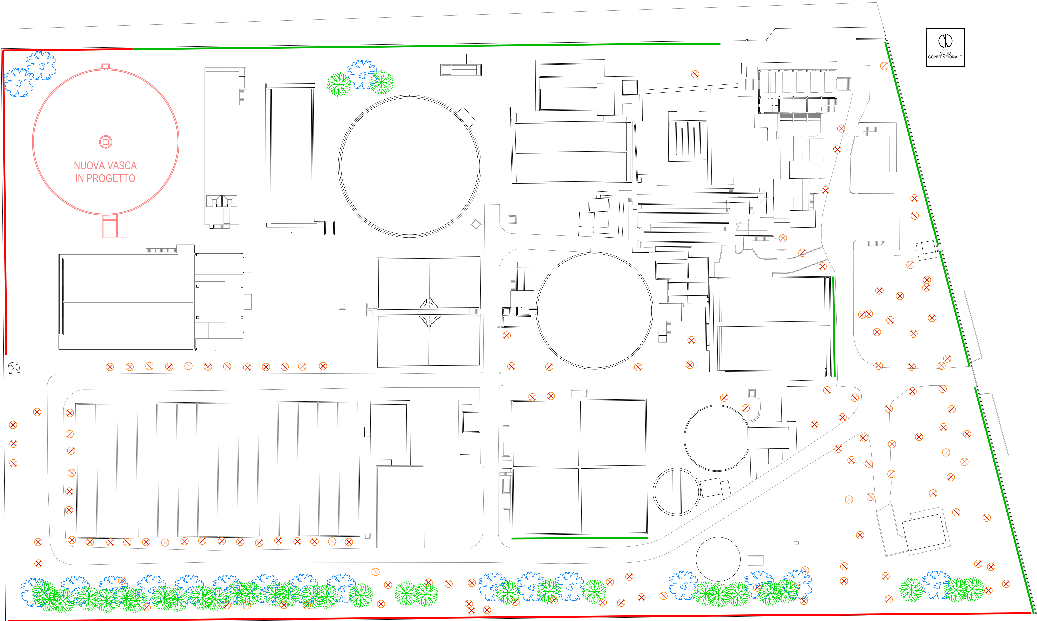
PLANIMETRIA IMPIANTO CONSORTILE DI DEPURAZIONE
